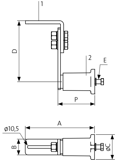
1. Halterung 2. Rosta-Element
